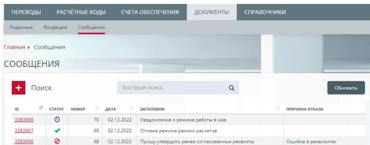
Рисунок 11-3 Окно «Сообщения»
