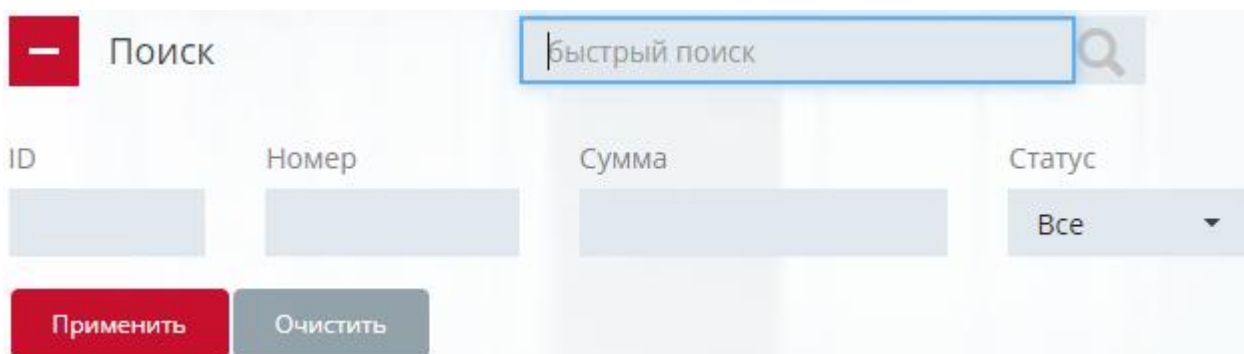
Рисунок 5-4 Вид фильтра
